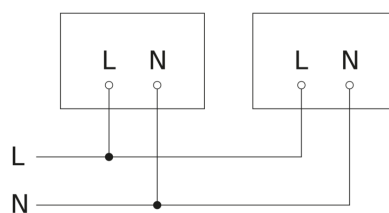
Diagrama electrónico interconexión maestro-maestro
